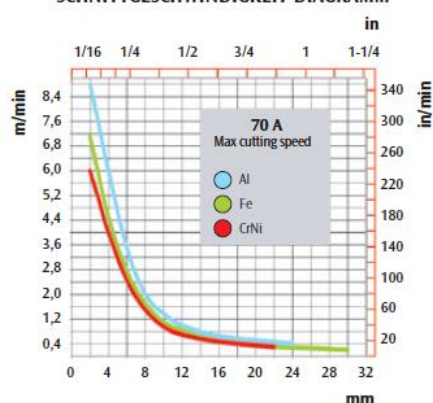
SCHNITTGESCHWINDIGKEIT-DIAGRAMM
